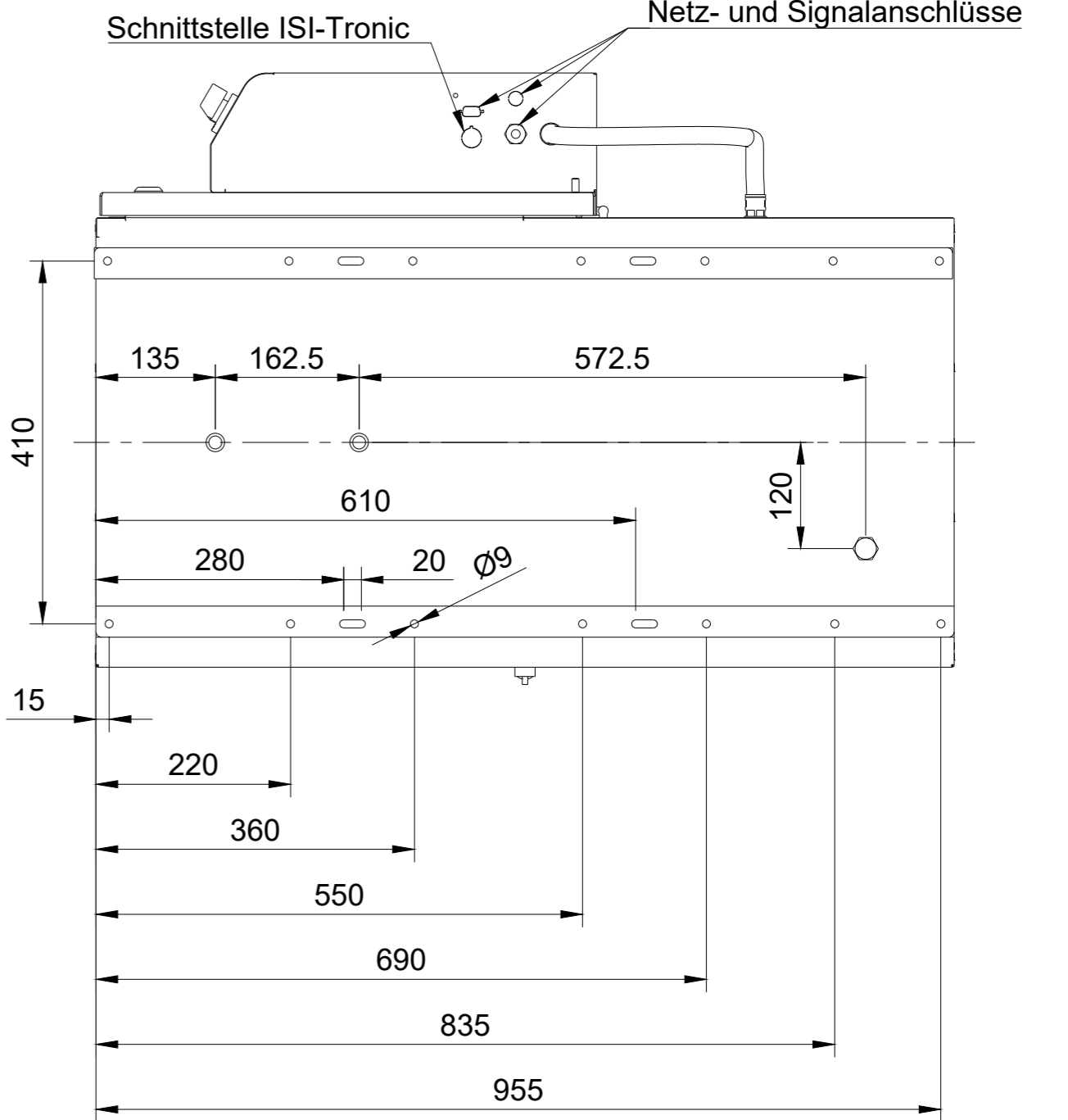
Ansicht A
