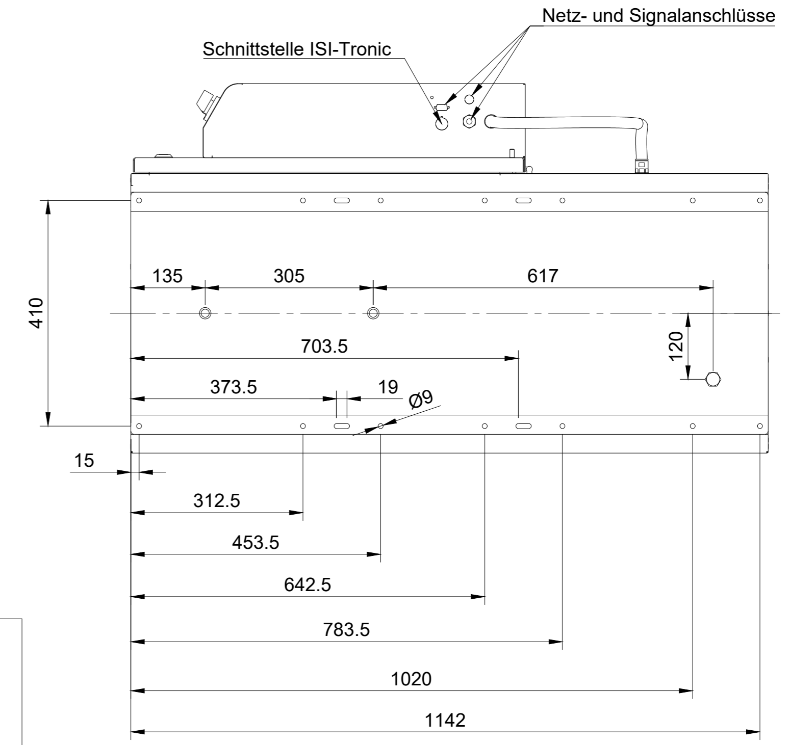
Ansicht A
