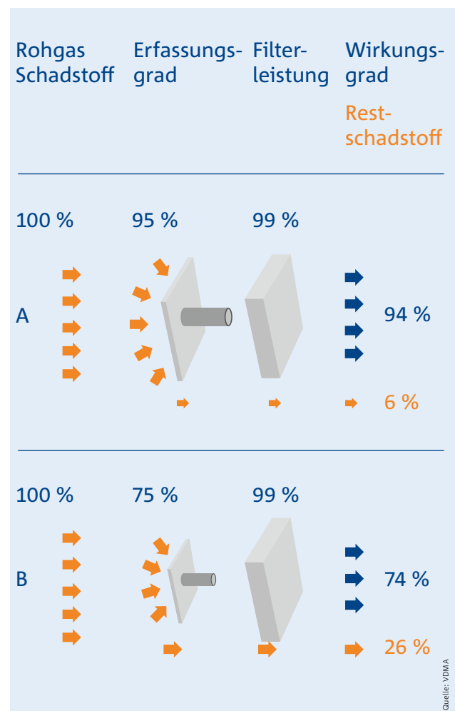
Einfluss des Erfassungselement-Abstandes auf die erforderliche Luftleistung
