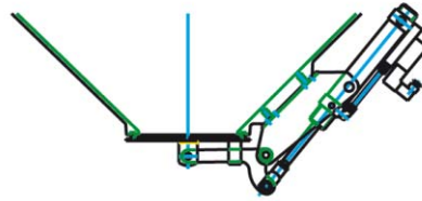
Elektropneumatische Klappe für DS 1...- Siloeinheiten, vacuumdicht
