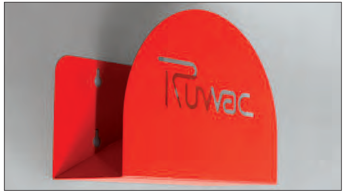
Schlauchhalter, Stahlblech, pulverbeschichtet, rot, Montage an der Wand L - 330 mm, B - 123 mm, H - 238 mm, incl. Befestigungsmaterial Art-Nr: 12080
