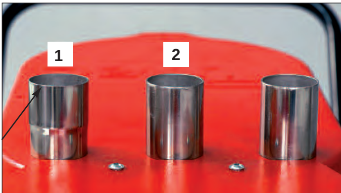
Zubehörhalter, Edelstahl, Montage auf der Schallhaube Höhe: 65 mm, für Zubehör 50 mm Ø 1. Innendurchmesser 50 mm - Art-Nr: 57121 2. Außendurchmesser 50 mm - Art-Nr: 54401
