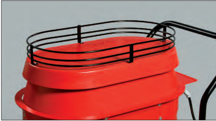
Zubehörkorb für W2 Stahlrohr pulverbeschichtet, schwarz, Montage auf der Schallhaube L - 578 mm, B - 324 mm, H - 70 mm Art-Nr: 16956
